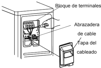
Diagrama de interconexión de las unidades Solo Frío (CO) , Frío Calor (HP)
